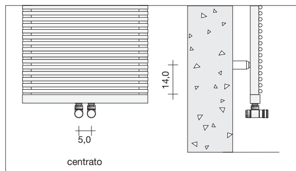
Schema tecnico allacciamento BA14 i5
